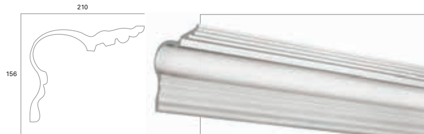
1K. Victorian Gutter
