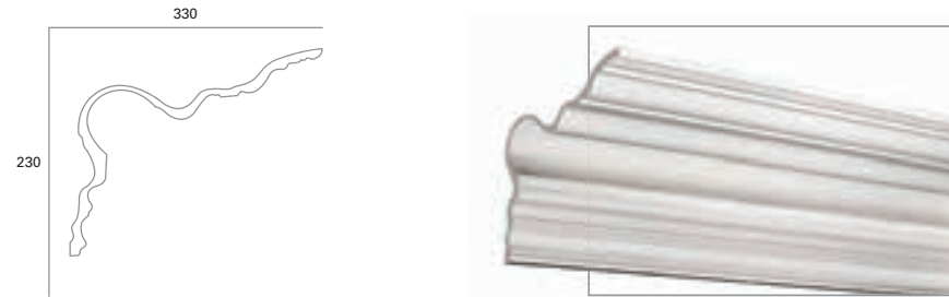
1E. Victorian Gutter
